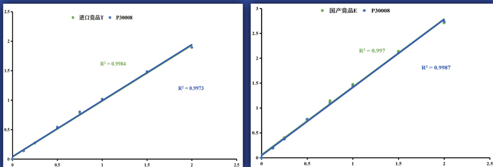
图1. P30008 与进口竞品T及国产竞品E 线性对比图
